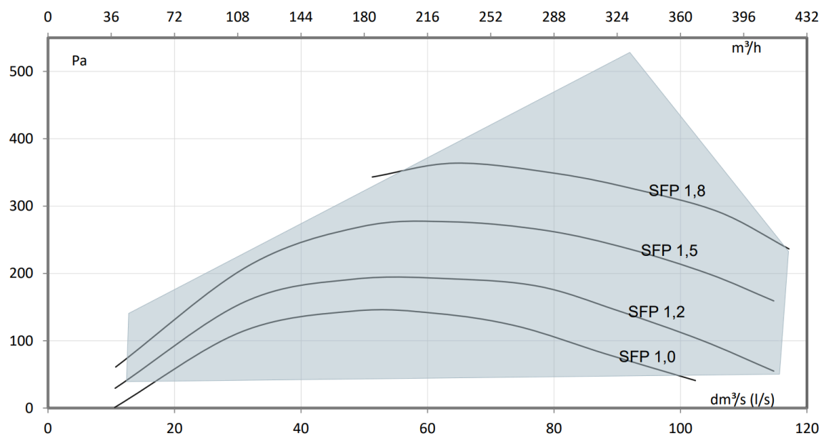
Rysunek 4. Strumienie powietrza nawiewanego i wywiewanego wentylatora, entalpiczny zespół wymiennika ciepła
