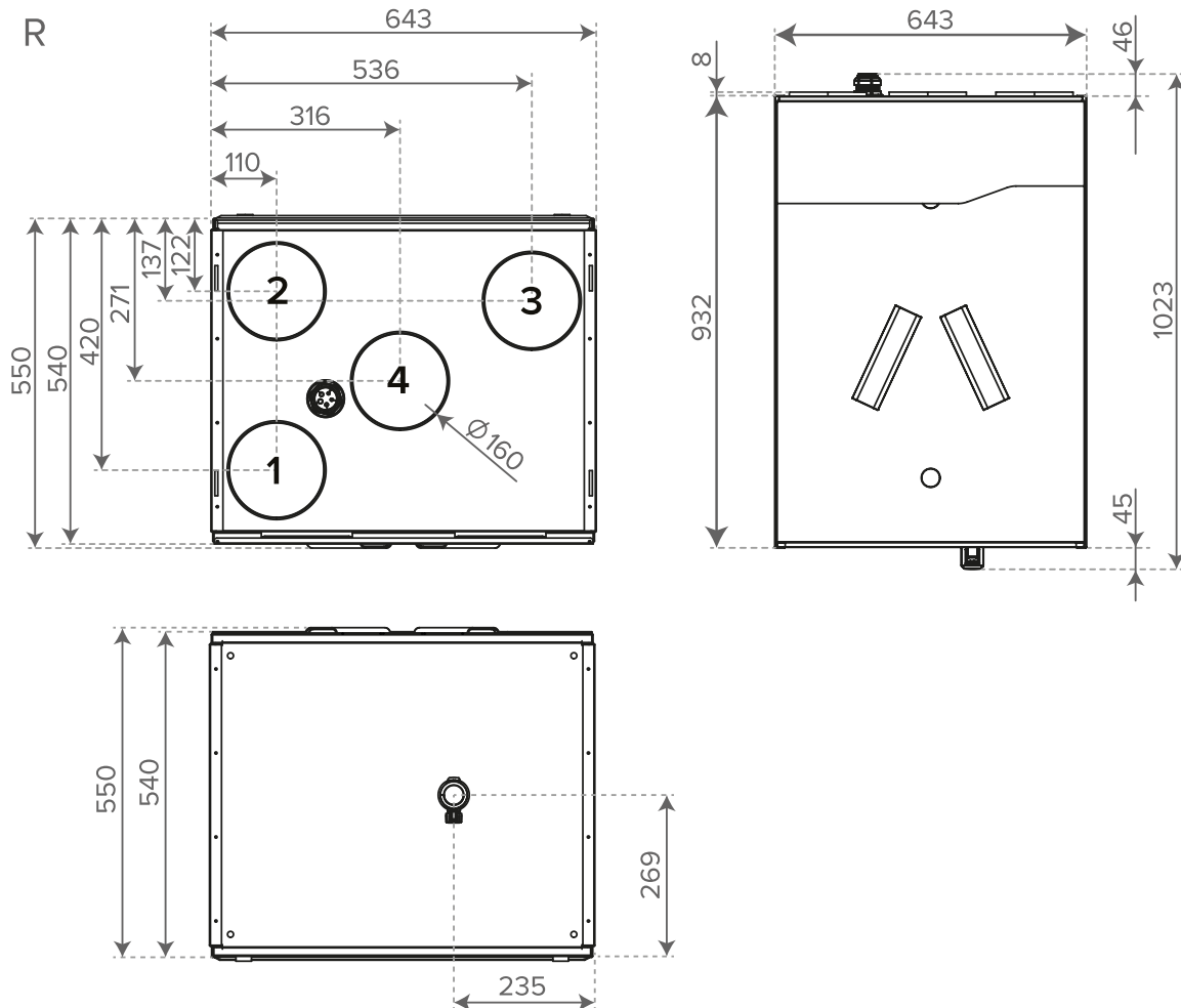
Rysunek 8. Wymiary oraz wyloty króćców Vallox 119 CFi L
